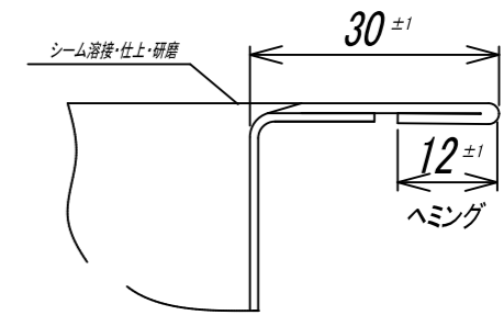
B-B断面 S=1/1
