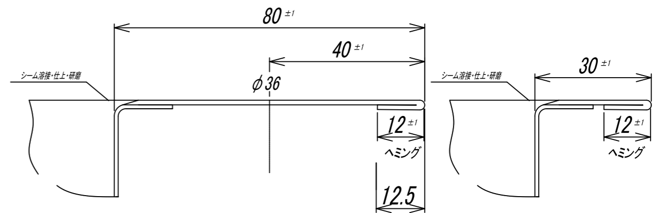
A-A'断面 S=1/1
